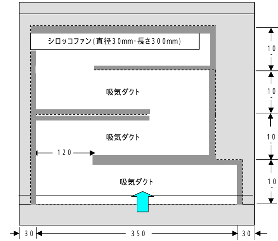
右側面図
