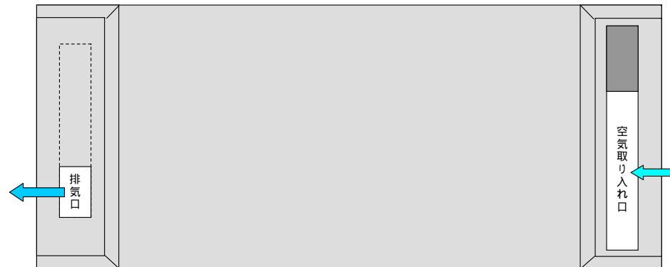
底部から見た図
