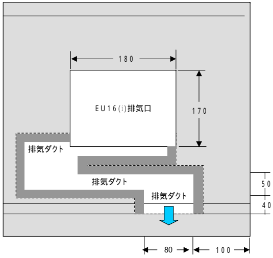
左側面図
